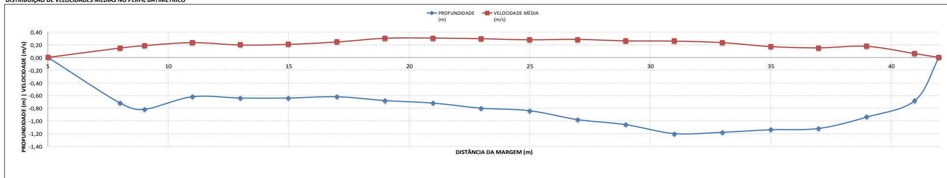
DISTRIBUIÇÃO DE VELOCIDADES MÉDIAS NO PERFIL BATIMÉTRICO
