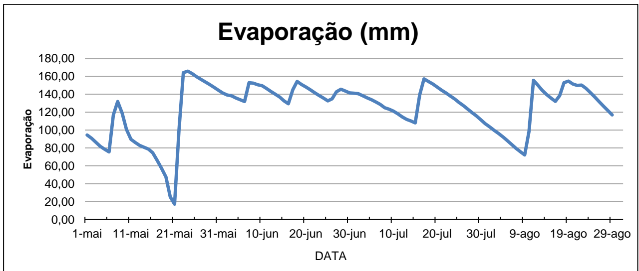
Gráfico 8 – Evaporação (mm) de 01 de maio a 31 de agosto - ano 2020.
