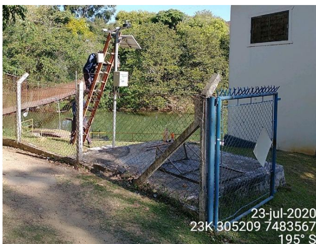
Foto 13 – Vista geral do trabalho de manutenção no PHJ – 10°C (Data: 23/07/20).
