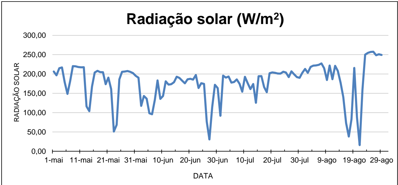
Gráfico 5 – Radiação Solar (W/m 2 ) de 01 de maio a 31 de agosto - ano 2020.
