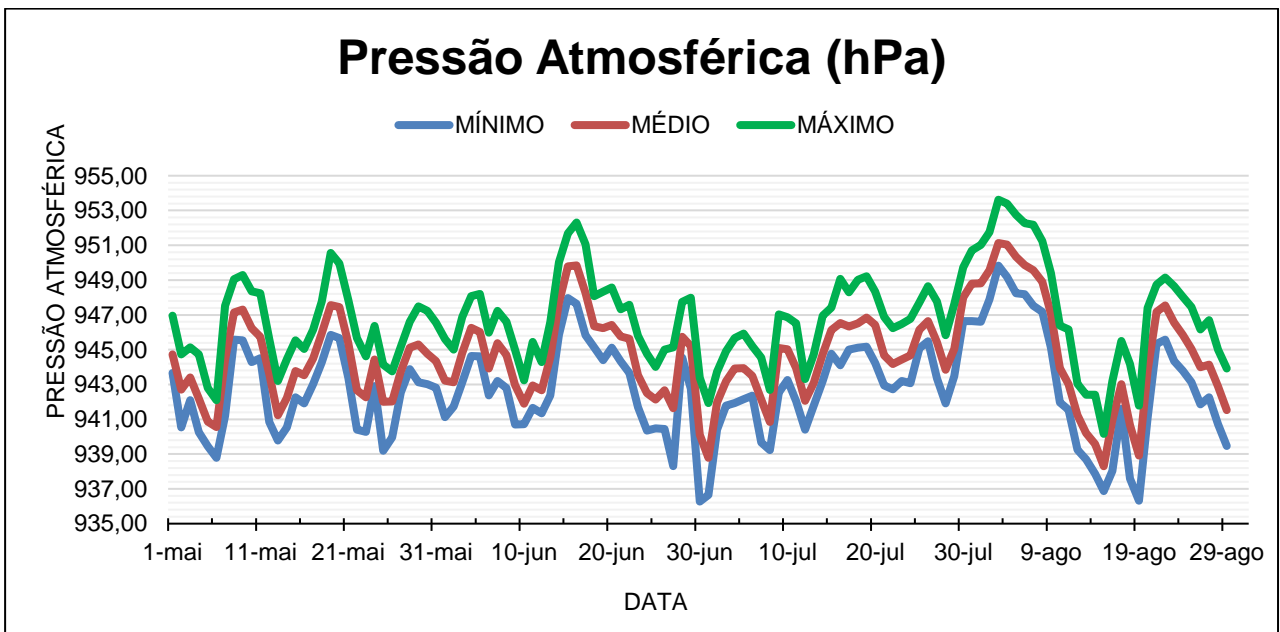
Gráfico 4 – Pressão Atmosférica (hPa) de 01 de maio a 31 de agosto - ano 2020.
