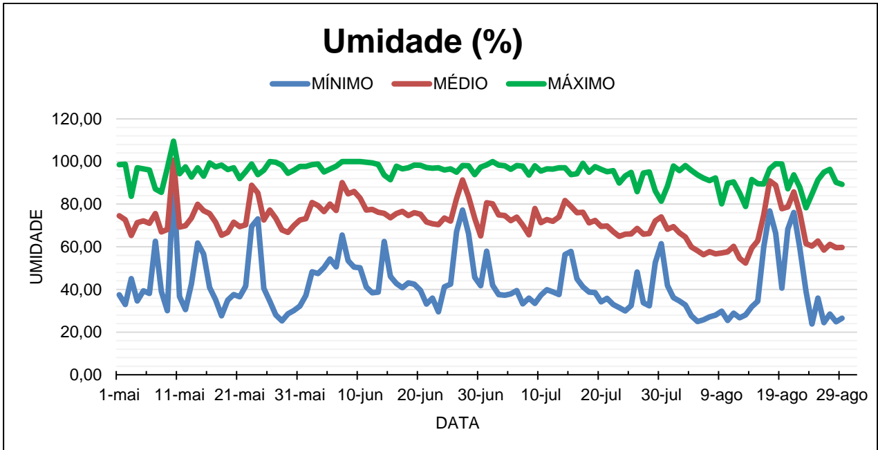
Gráfico 3 – Umidade (%) de 01 de maio a 31 de agosto - ano 2020.
