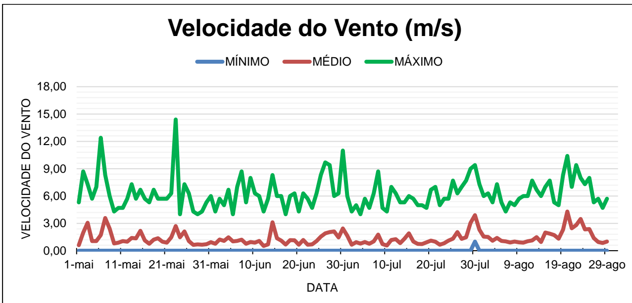
Gráfico 6 – Velocidade do Vento (m/s) de 01 de maio a 31 de agosto - ano 2020.
